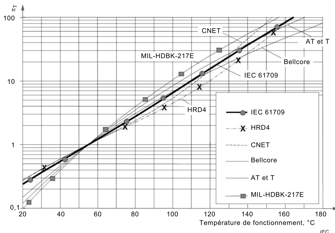
Figure 1 – Comparaison des facteurs \pi_T traduisant l'influence de la température pour les circuits intégrés CMOS
