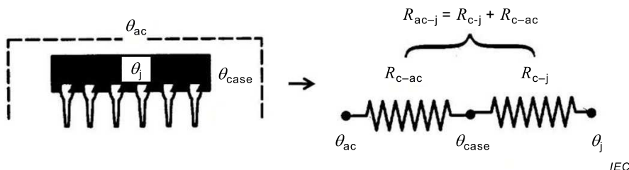
Figure B.2 – Modèle de résistance thermique
